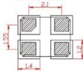
推荐使用焊盘
