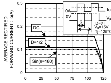
CASE TEMPARATURE : T_c(°C) Derating Curve*( I_o - T_c )
