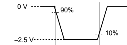
(b) V_{IN}
